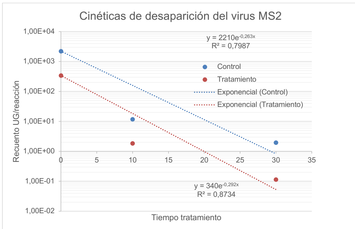
Figura 1. Cinéticas comparadas de desaparición del virus MS2.
