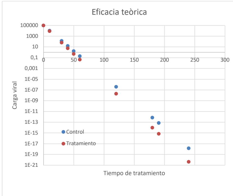
Figura 2. Cinètica teòrica de eliminaci3n del virus en condicions control i de tractament. El diferencial de taxa genera una eficàcia de resposta que augmenta amb el temps (tabla 3)
